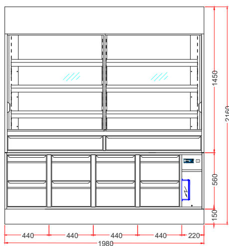
KKV 198-E R290 SANS GROUPE AVEC TIROIR
