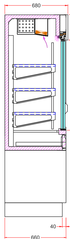
KKV sans groupe avec tiroir
