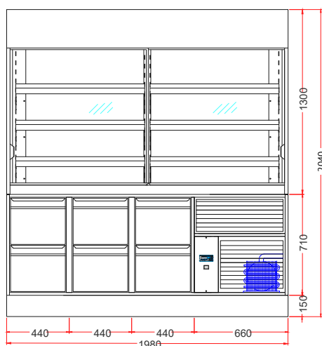
KKV 198-E R290 GROUPE LOGE SANS TIROIR
