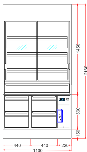
KKV 110-Z SANS GROUPE AVEC TIROIR
