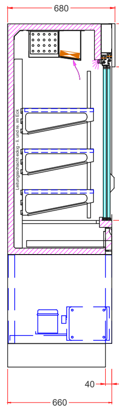
KKV groupe logé avec tiroir
