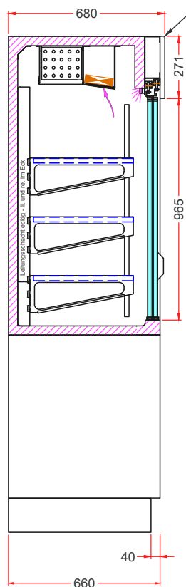
KKV sans groupe sans tiroir
