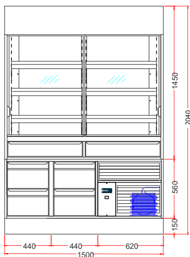
KKV 150-E R290 GROUPE LOGE AVEC TIROIR
