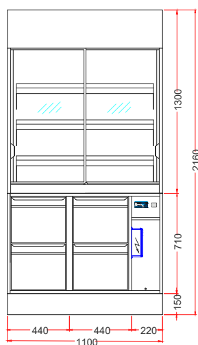
KKV 110-Z SANS GROUPE SANS TIROIR
