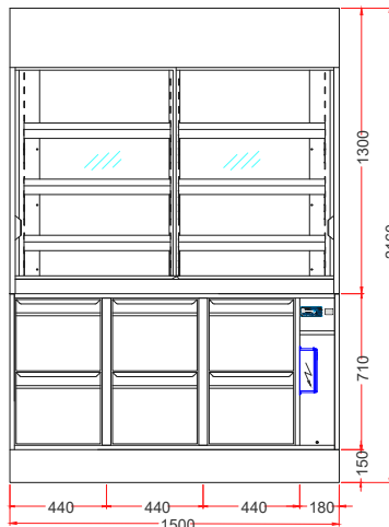
KKV 150-Z SANS GROUPE SANS TIROIR
