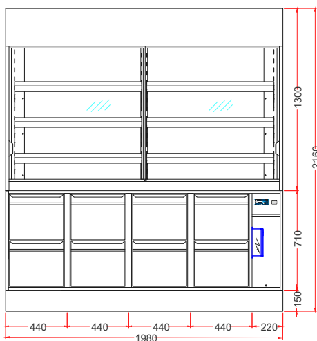
KKV 198-Z SANS GROUPE SANS TIROIR
