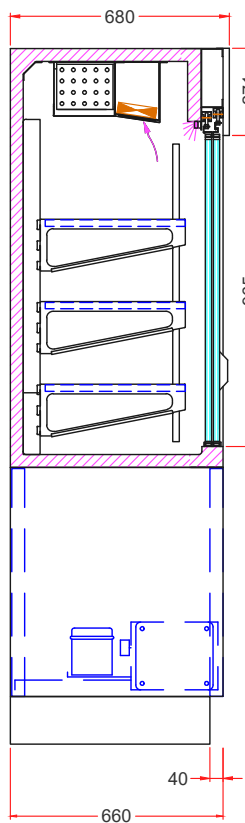
KKV groupe logé sans tiroir
