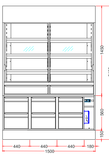
KKV 150-Z SANS GROUPE AVEC TIROIR
