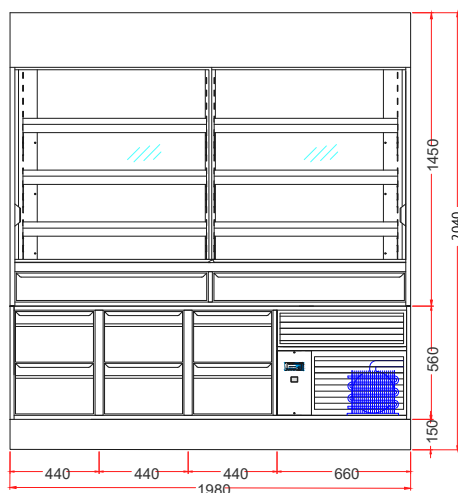
KKV 198-E R290 GROUPE LOGE AVEC TIROIR
