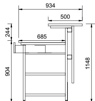
> Eyota caisse d'angle de coin E90R
