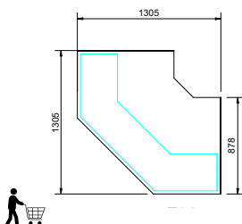
> Eyota caisse d'angle E90D
