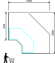
> Eyota caisse d'angle E90I
