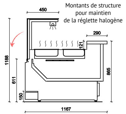
> Enixe K 450 (H Combi)
