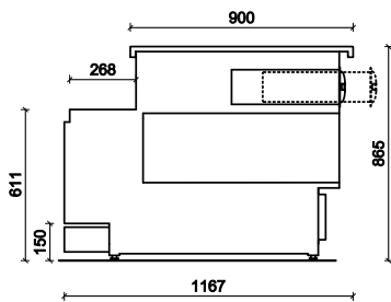
> Enixe K caisse standard
