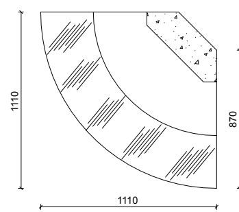
AEC 90 Angle arrondi 90° ext.
