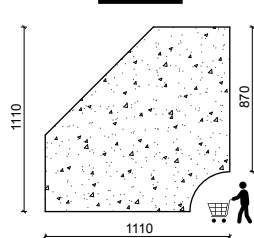
AIC90 Angle arrondi 90° int. caisse std
