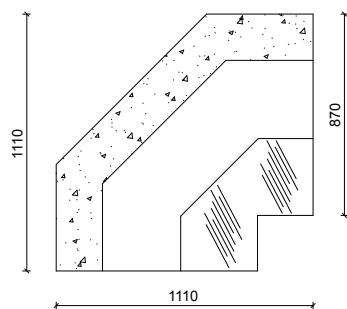
AIR 90 Angle pans coupés 90° int.
