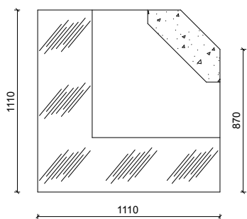
AER 90 Angle pans coupés 90° ext.
